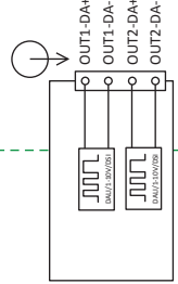
DGBM200 2 CH Driver module
