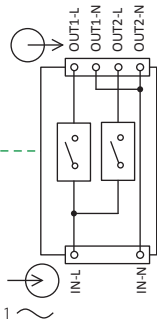
DGRM204 2 x 4 A relay module
